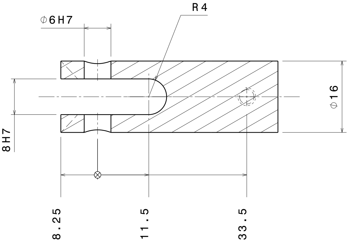
CORTE T-T
