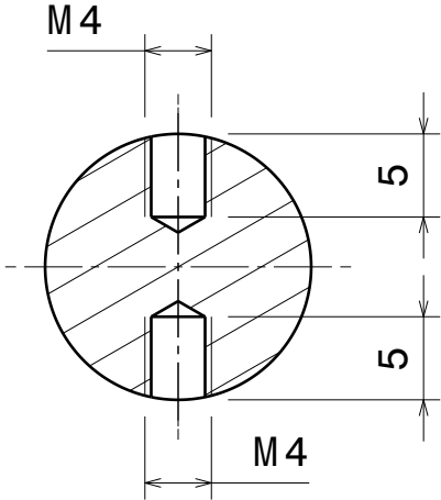
CORTE S-S
